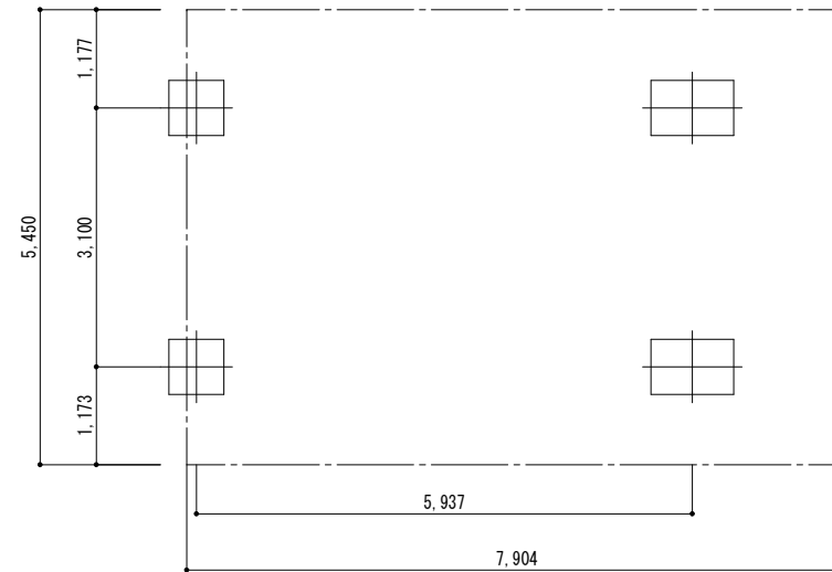
■基礎配置図
